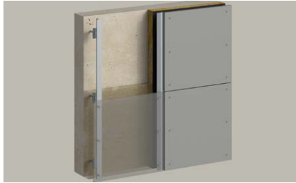
Facciate ventilate
